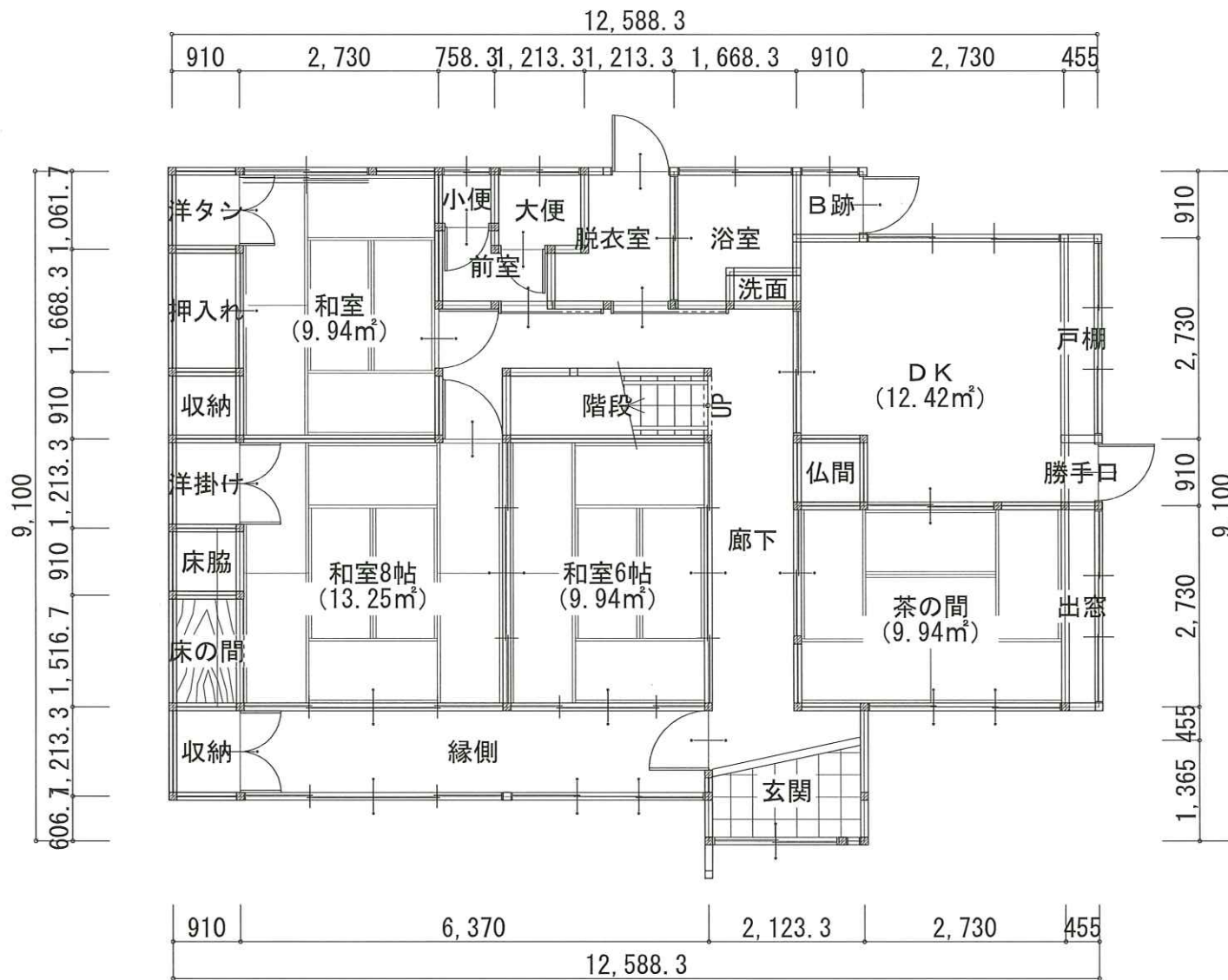
改修前 既存図面
